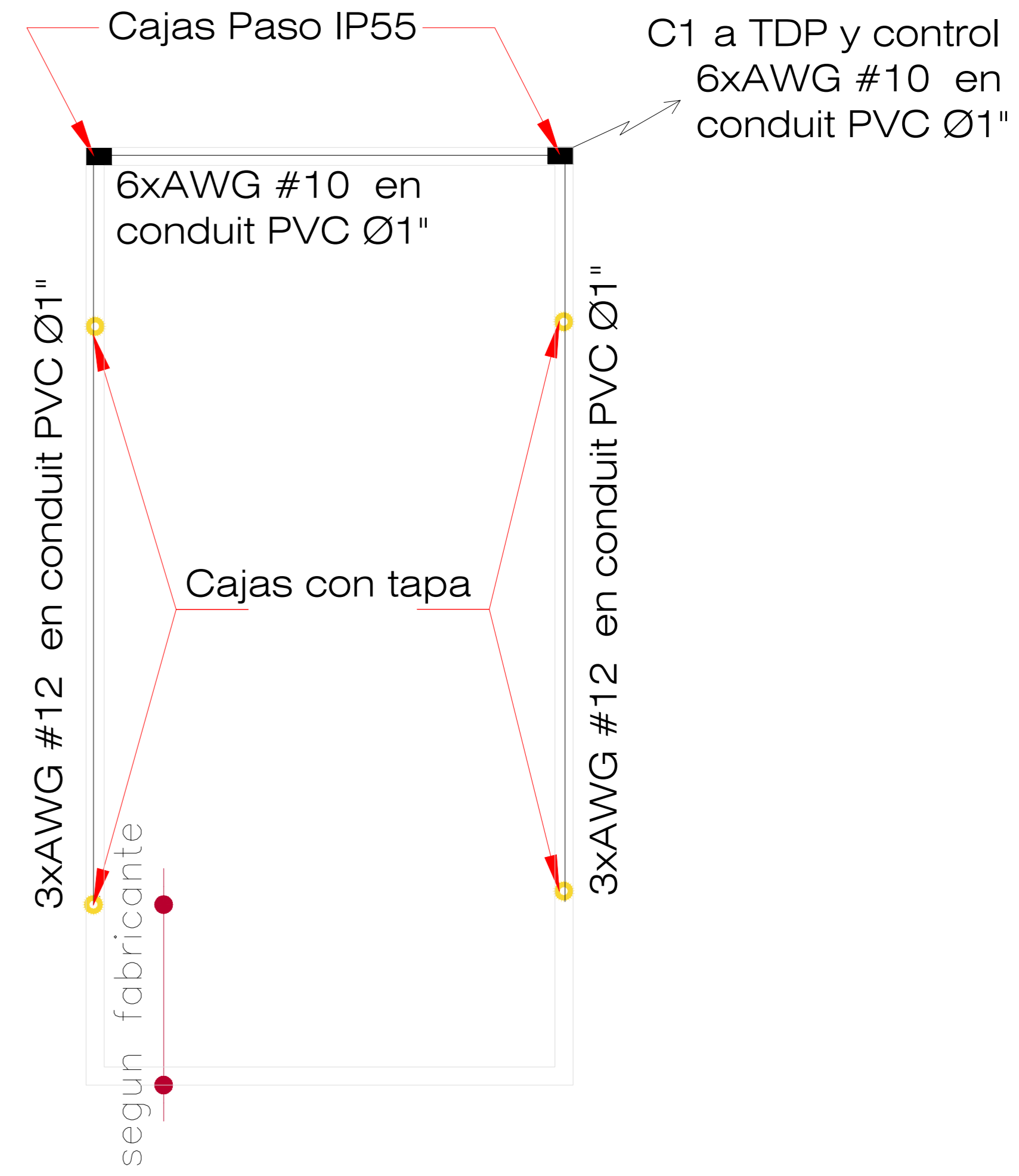
CANCHA DE PADEL INSTALACIÓN ELÉCTRICA Escala 1:200
