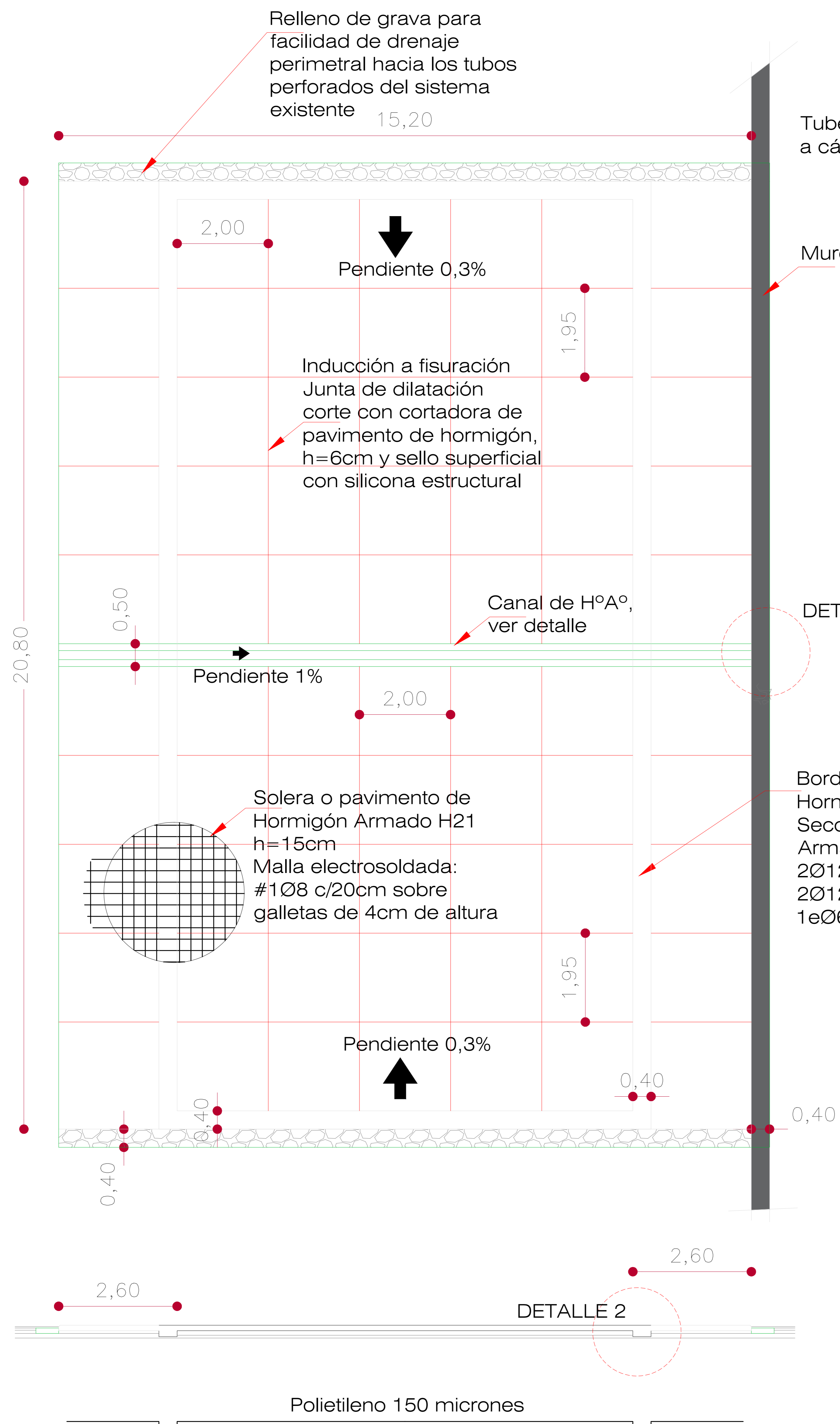
CANCHA DE PADEL ESTRUCTURA Y DETALLES PLATAFORMA Escala 1:100
